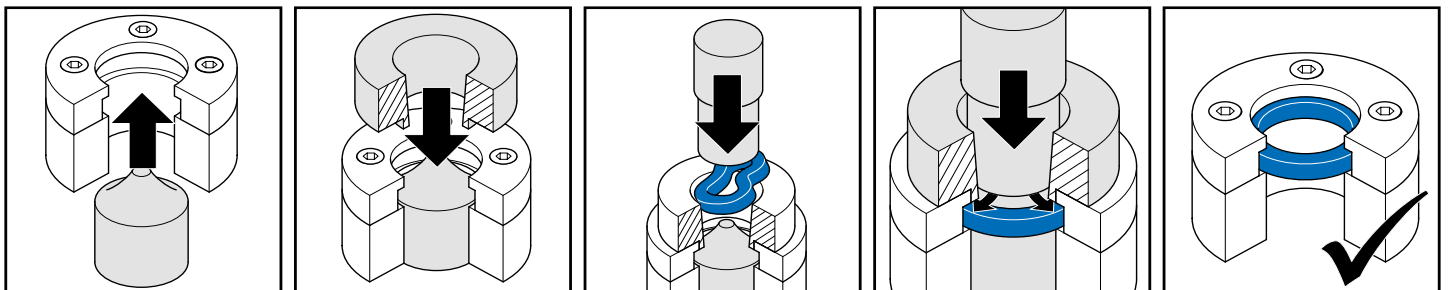
1B. Fitting with Pusher, cone sleeve and stops | Montage avec mandrin, douille conique et contre-appui | Construído com Pusher, manga cono y paras | Construído com Pusher, cone manga e batente
